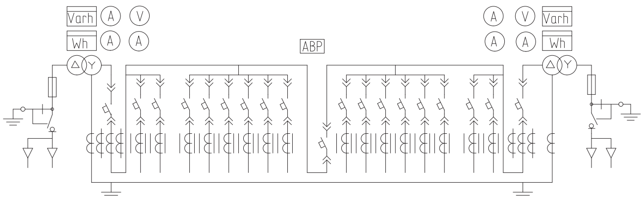
Однолинейная принципиальная схема КТСП
