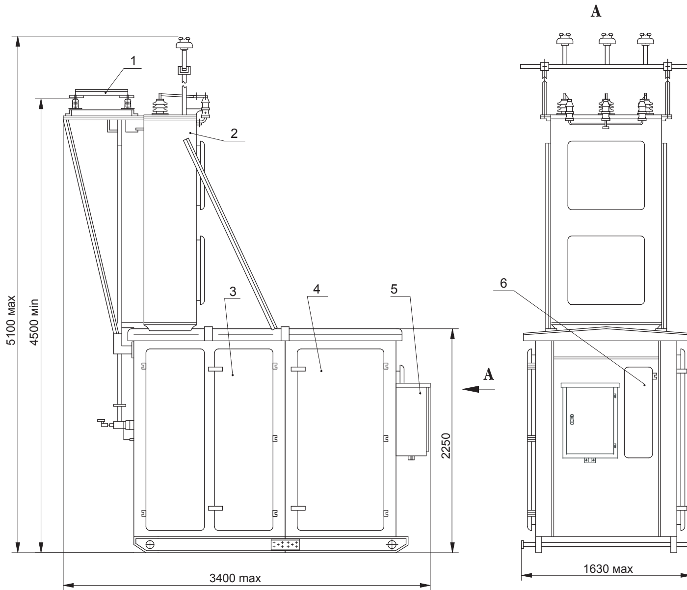
Габаритные размеры и масса КТППН-82, КТППН-05
