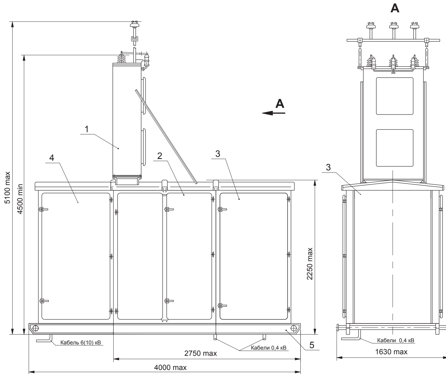
Габаритные размеры и масса КТПТАС с КУ
